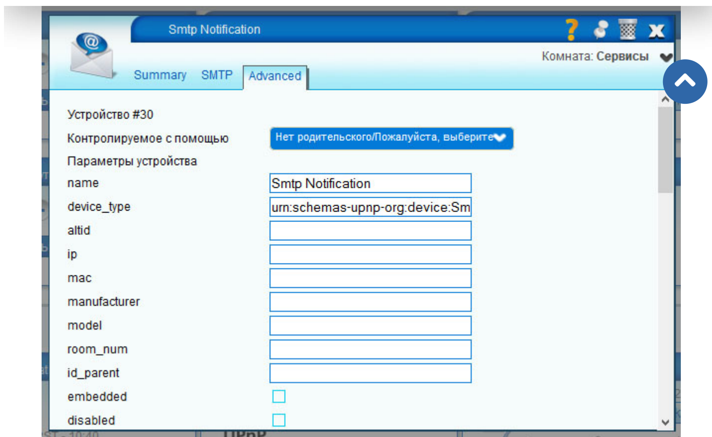
Рис. 3. Дополнительное окно настройки «eMail Notification», откуда надо взять номер устройства, в данном случае это номер 30
